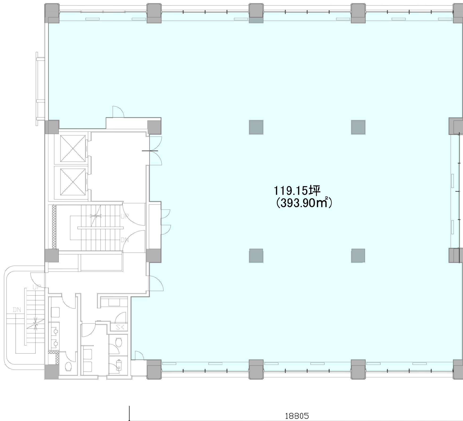
物産ビル 3階建築平面図
